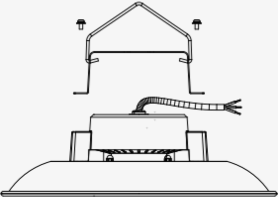
锁支架
