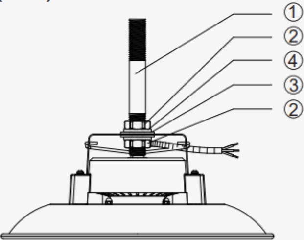
锁好支架后，再安装吊杆
