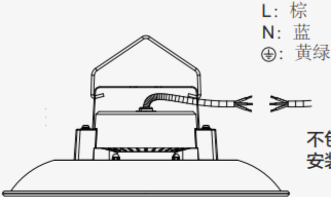
接线
