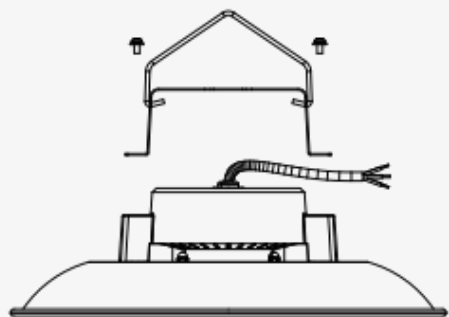
1. 锁支架;
