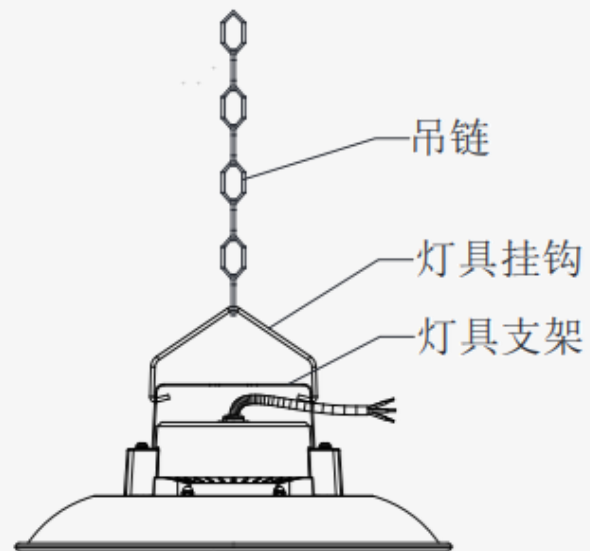
4. 灯具挂钩回挂支架侧孔
